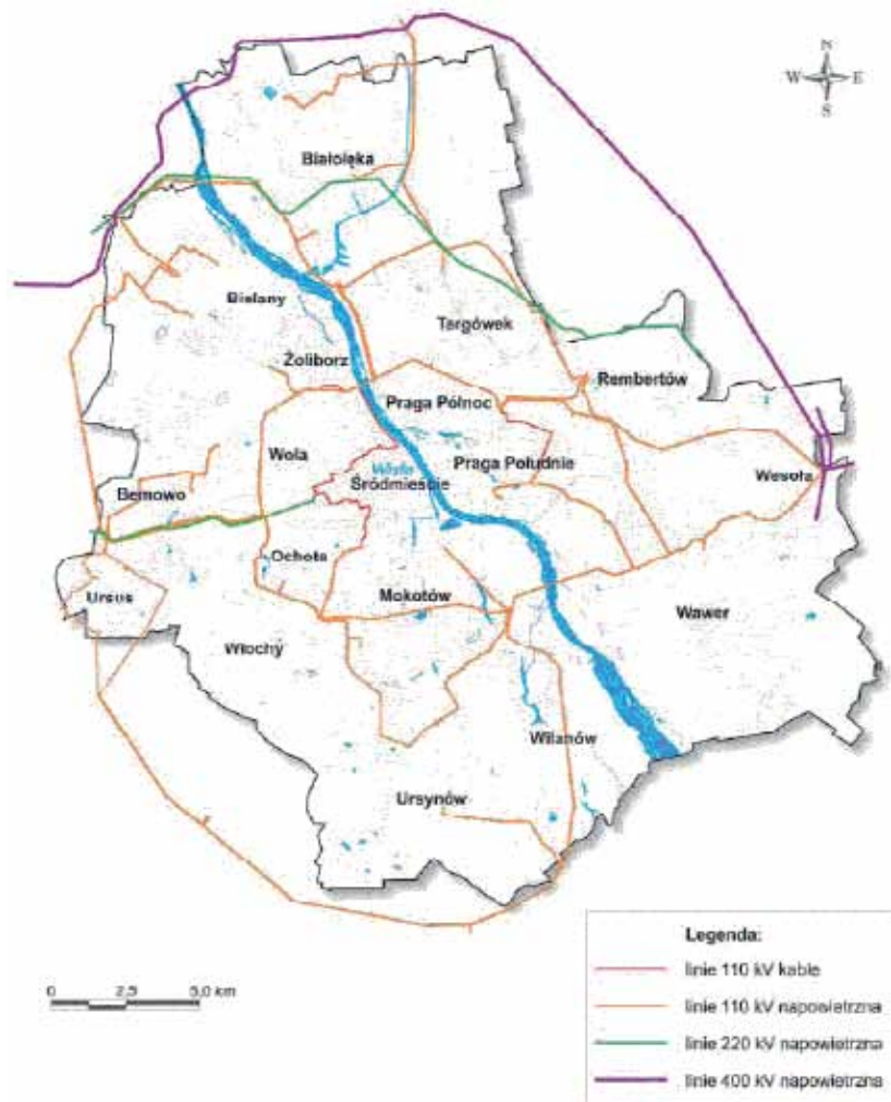
Rysunek 19. Rozkład linii elektroenergetycznych w Warszawie
