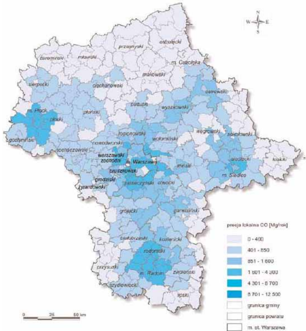
Rysunek 14. Lokalna presja tlenku węgla w województwie mazowieckim w 2004 r.
