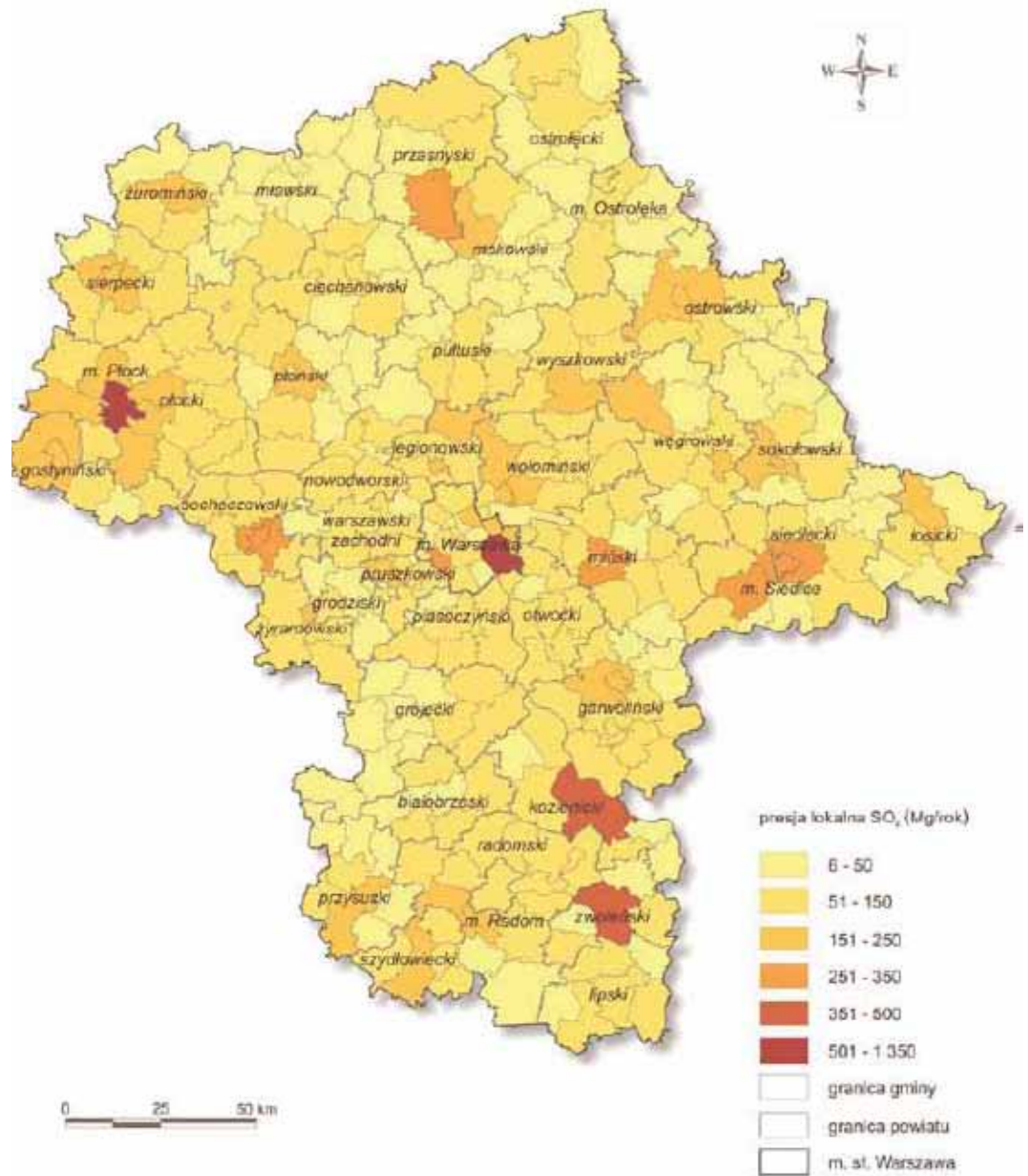
Rysunek 12. Lokalna emisja dwutlenku siarki w województwie mazowieckim w 2004 r.
