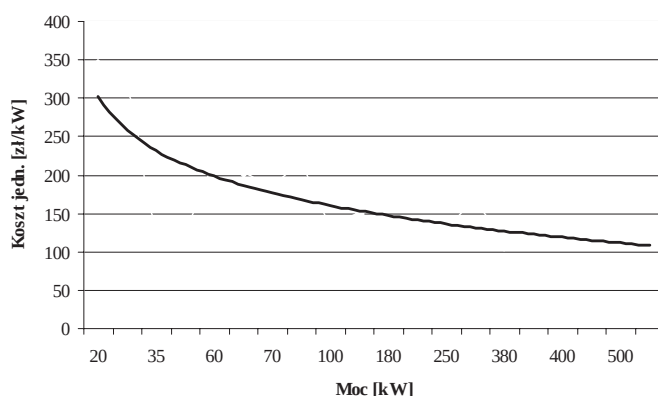
Rys. 8 Jednostkowe koszty zakupu kotłów na słomę
