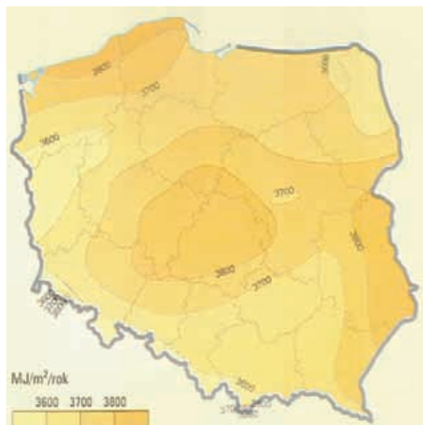
Rys. 4 Roczne całkowite promieniowanie w Polsce
