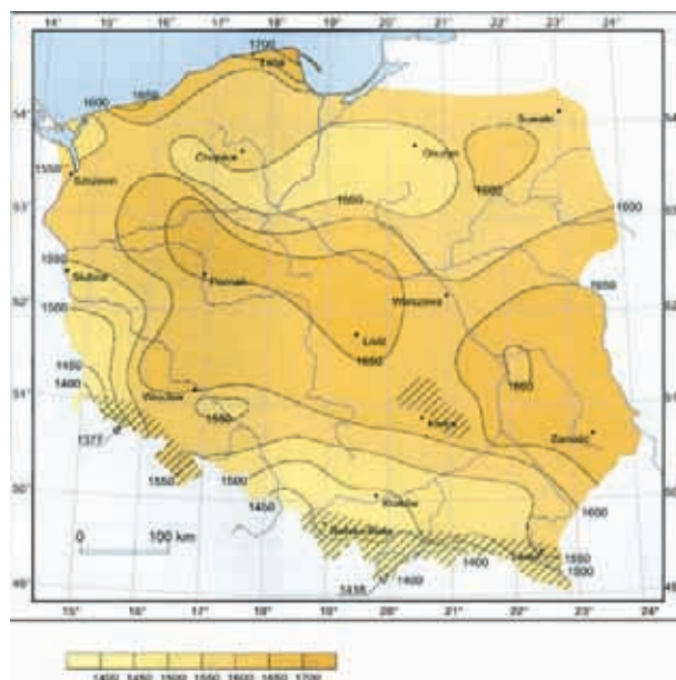
Rys. 3 Średnioroczne sumy nasłonecznienia w godzinach
